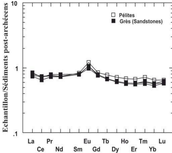
Figure 7. Spectres des Terres Rares des métasédiments de Kalana normalisés aux sédiments post-archéens (Taylor &amp; Mc Lennan 1985).
