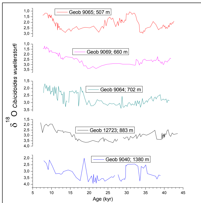
Figure 4. \delta^{18}\text{O} values of benthic foraminifera ( Cibicoides wuellerstorfi ).
