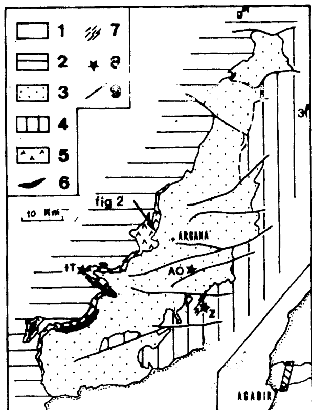
Figure 1 : Affleurements des roches volcaniques dans le couloir d'Argana (d'après MEDINA & EL AMRANI, 1989, complété d'après AMRHAR, 1989).
