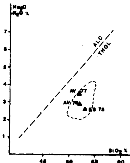
Figure 4 : Position des échantillons AV76, AV77 et ES75 (analyses in MANSPEIZER & al., 1978) dans le diagramme Na 2 O + K 2 O = f(SiO 2 ) de Kuno (1950). En tirets : champ des laves triasiques de l'Atlas de Marrakech (TANE & al., 1983).
