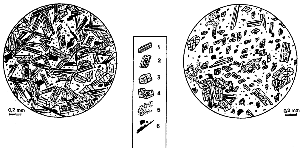
1 : plagioclase; 2: idem. altéré 3: clinopyroxène; 4: idem. altéré; 5: chlorite; 6: opaque
