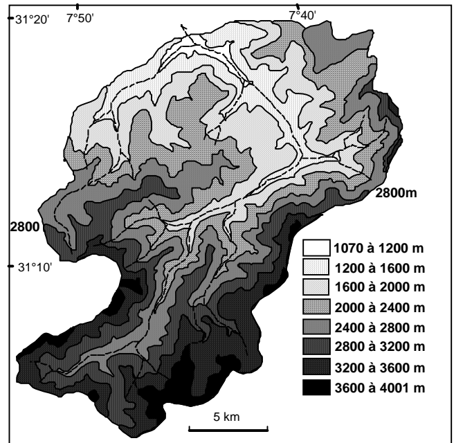
Figure 5. Hypsométrie du bassin versant de l'Ourika à Aghbalou.
